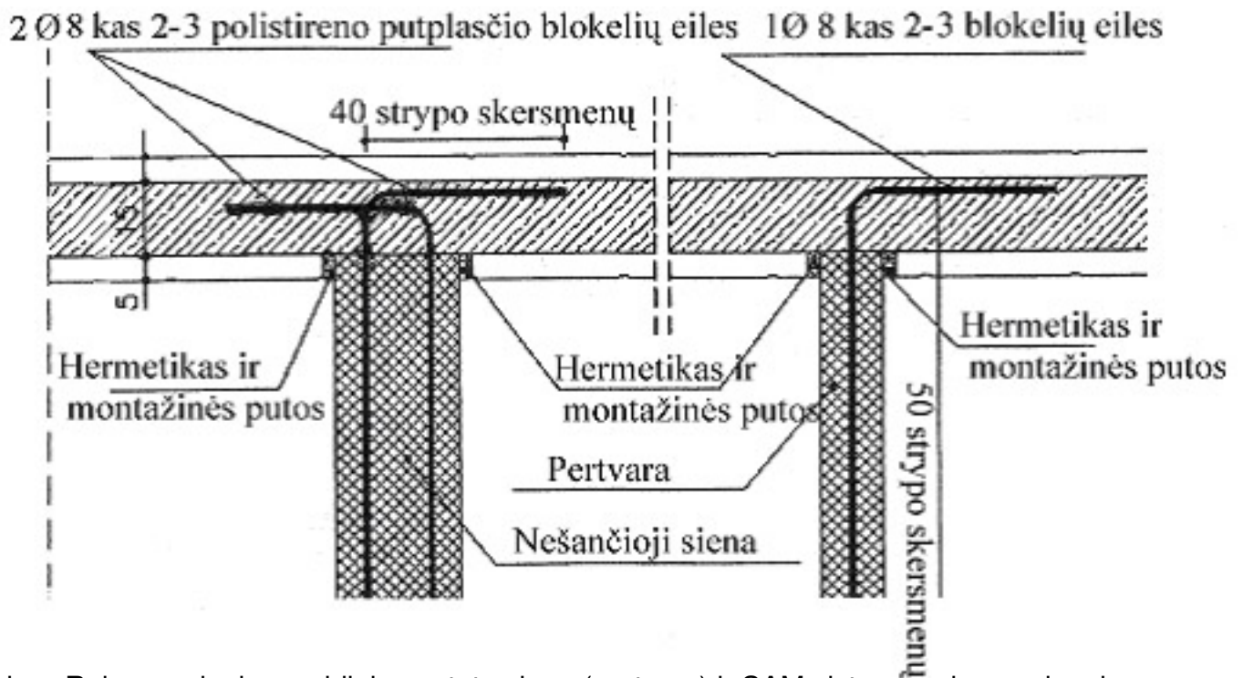
Schem. Rekomenduojama vidinių pastato sienų (pertvarų) ir SAM sistemos sienų sujungimo
